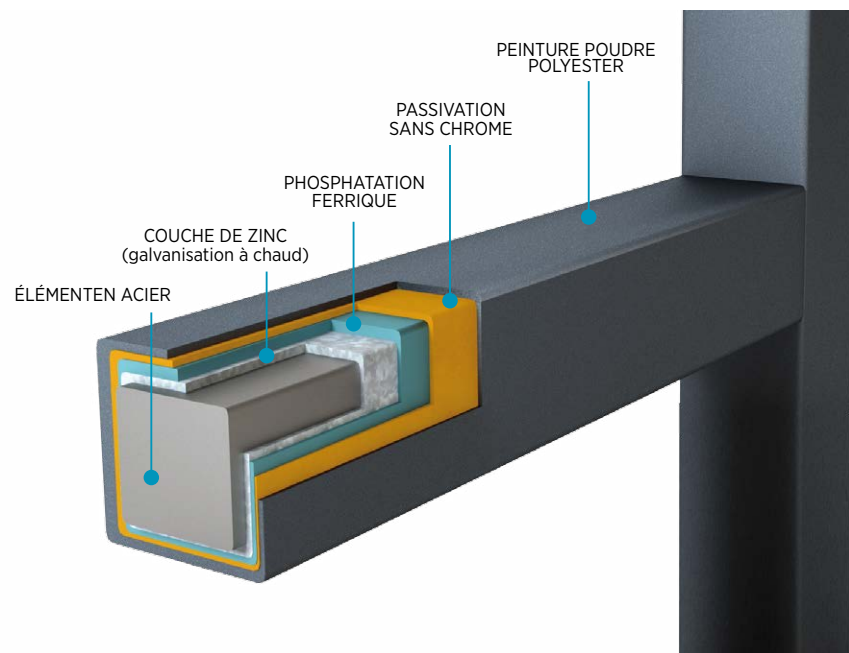
Coupe d'un élément protégé dans le système DUPLEX
